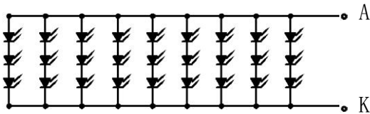
LED 电路图
